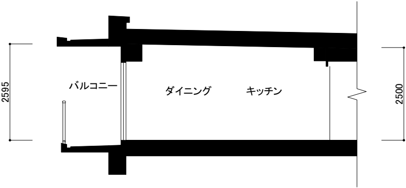
ダイニング、キッチン断面
