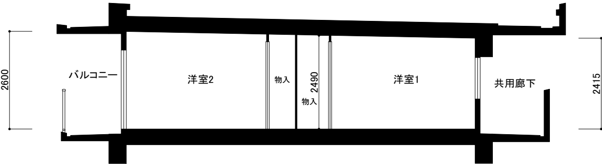
洋室1、2断面
