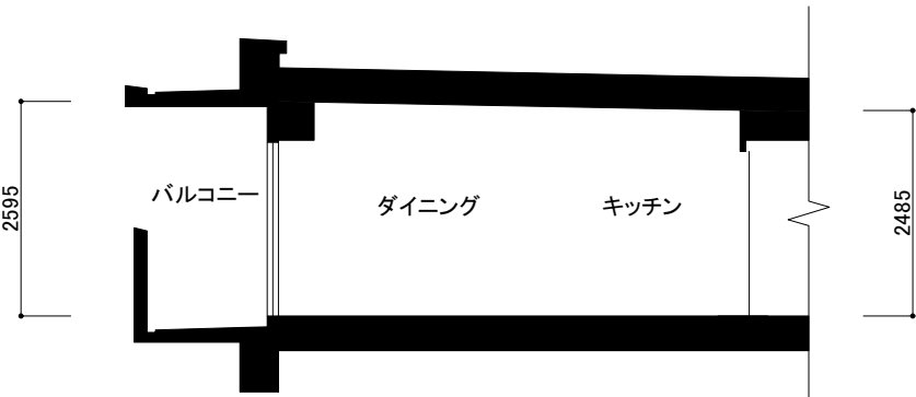
リビング・ダイニング、キッチン断面
