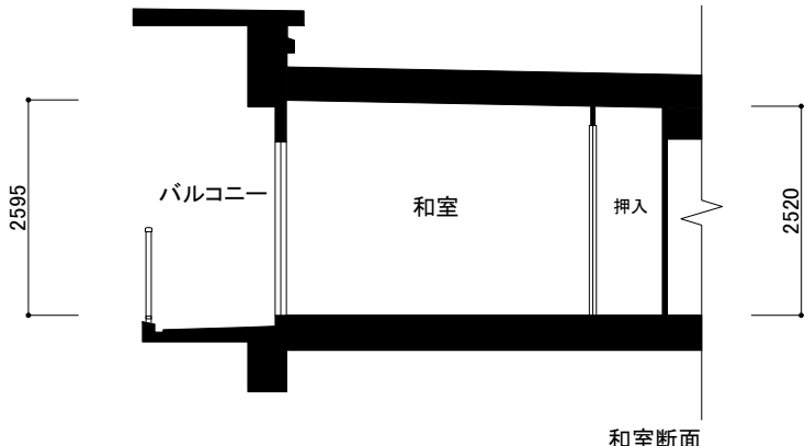
和室断面
