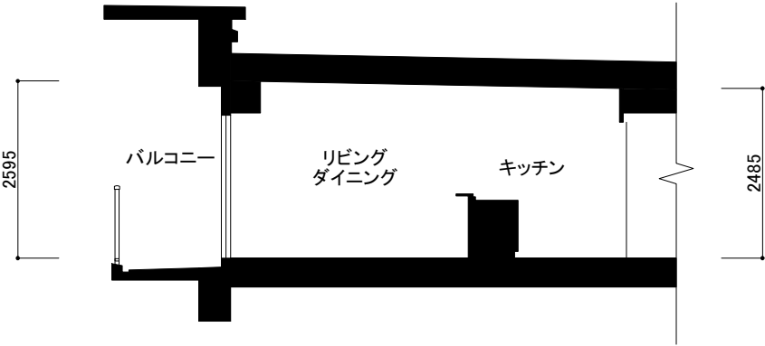
リビング・ダイニング、キッチン断面
