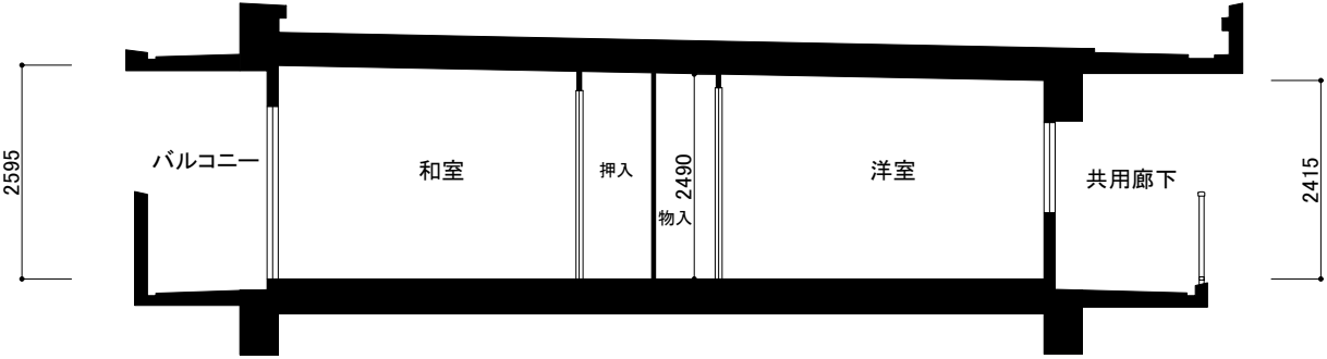
和室、洋室断面
