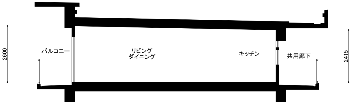
リビング・ダイニング、キッチン断面
